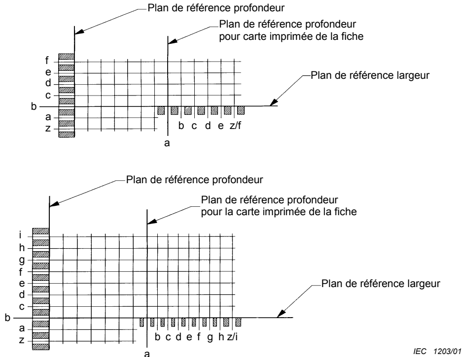
Figure 1 – Implantation typique de grille pour modules de connecteurs de 2,0 mm
