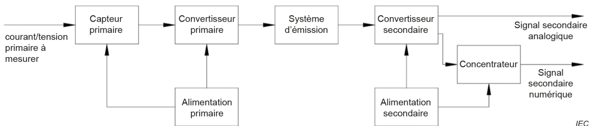
Figure 1 – Schéma fonctionnel général des LPIT monophasés
