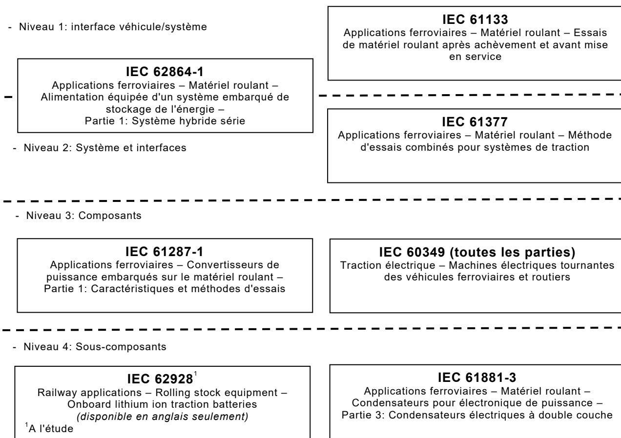
Figure 1 – Hiérarchie des normes associées à l'IEC 62864-1
